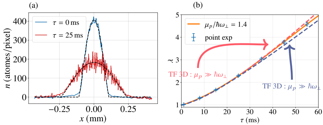
FIGURE 5.4 – (a) Profil de densité à l’équilibre dans le piège harmonique longitudinal (bleu), ajusté par n_0(x) selon Eq. (5.32) (noir pointillé). La courbe rouge montre le profil après une expansion longitudinale \tau = 25 ms, avec un facteur d’échelle \lambda extrait en ajustant le profil par une courbe homothétique à la densité initiale (noir pointillé), cf. Eq. (5.7). (b) Points bleus : facteurs d’échelle \lambda(\tau) extraits expérimentalement. Courbe orange : résultats numériques obtenus en résolvant les équations hydrodynamiques (Eq. (5.29)) avec \mu_p/\hbar\omega_\perp = 1.4 . Les courbes pointillées montrent les évolutions attendues de \lambda en résolvant Eq. (5.19) pour \alpha = 1 (TF 1D) et \alpha = 1/2 (TF 3D).
