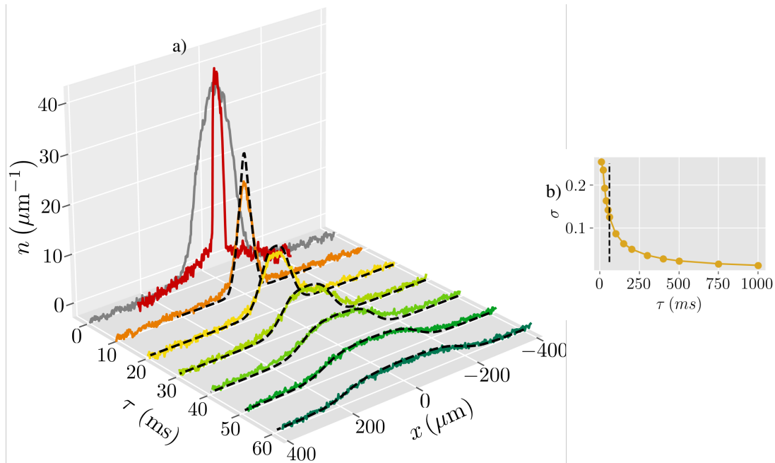
FIGURE 5.8 – (a) La tranche, centrée en x_0 = 0 \mu\text{m} , subit une expansion le long de l’axe longitudinale d’une largeur \ell = 37 \mu\text{m} . Le profil initial du gaz est montré en gris. Les variations de densité pour différents temps d’expansion sont représentées par des courbes colorées. Les lignes pointillées noires indiquent les résultats des simulations GHD pour une distribution de rapidités initialement thermique, paramétrée par la température T et le potentiel chimique \mu(x_0) = \mu , tels qu’ils sont extraits du profil de densité in situ. (b) L’écart-type \sigma(\tau) (Eq. (5.33)) est calculé entre la distribution de rapidités et les résultats des simulations GHD en fonction du temps d’expansion \tau . La ligne verticale noire correspond au temps d’expansion utilisé dans l’expérience.
