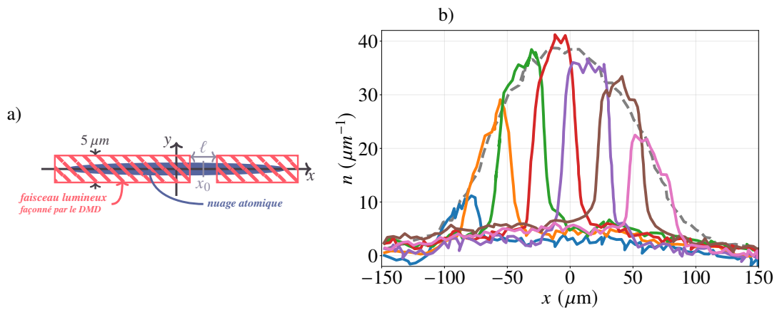
FIGURE 5.5 – (a) Schéma illustrant la sélection d'une région du nuage atomique, ici représentée par un ellipse bleu illuminé par un faisceau modulé à l'aide du DMD.
