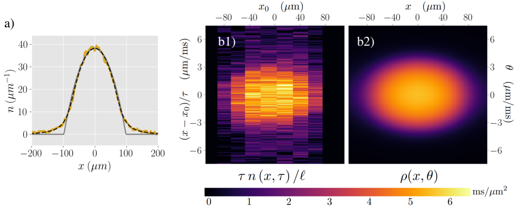
FIGURE 5.6 – a) Profil de densité d’un nuage atomique initialement à l’équilibre dans un piège harmonique avec \omega_{\perp} = 2\pi \times 2.6 kHz et \omega_{\parallel} = 2\pi \times 5 Hz (zone en jaune). La courbe grise représente le profil parabolique attendu à l’état fondamental dans le régime qBEC, décrit par l’équation d’état n(x) = [\mu - V_{\parallel}(x)]/g . La courbe noire en pointillés correspond à un ajustement des données expérimentales en supposant que le système soit bien décrit par un ensemble thermique (TBA (Sec 2.2.2)). Cet ajustement permet d’extraire une température T = 90 nK et un potentiel chimique \mu/k_B = 49 nK. (b1) Profils de densités pour différents centres de sélection x_0 représentés sur la Fig. 5.5(b). Les sélections sont de taille \ell = 37 \mu\text{m} et les profils obtenus après un temps d’expansion \tau = 40 ms. Pour comparer les résultats à une distribution de rapidités, les profils de densités sont multipliés par le rapport \tau/\ell et sont tracés en fonction de (x - x_0)/\tau (b2). (b2) Prédiction théorique de la distribution de rapidités spatialement résolue \rho(x, \theta) à l’équilibre thermique dans un potentiel harmonique longitudinal avec \omega_{\parallel} = 2\pi \times 5 Hz. La température T et le potentiel chimique \mu utilisés sont eux obtenus à partir du profil in situ (a).
